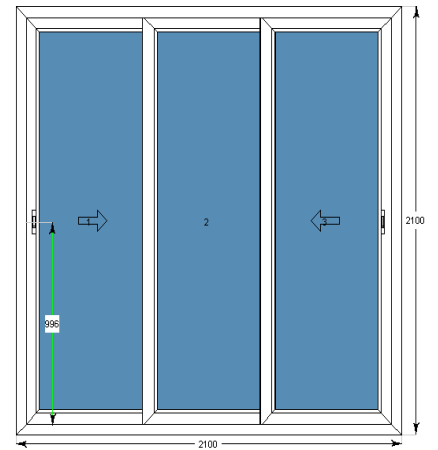
3 - Track Sliding Door
