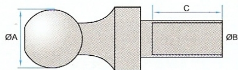
Hitch Ball
